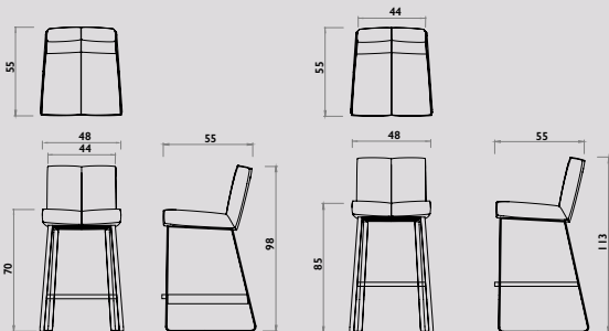
Noble keukenkruk
